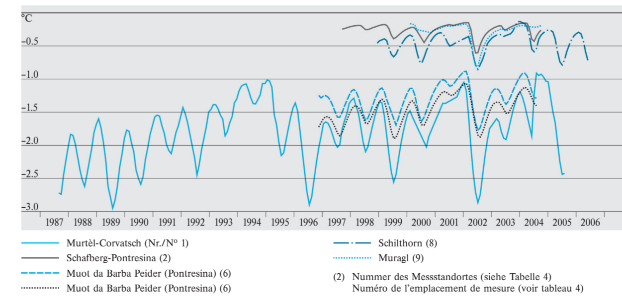
Fig. 6 Zeitreihen der Permafrosttemperaturen in ungefähr 10 m Tiefe Séries chronologiques des températures du permafrost à environ 10 m de profondeur
